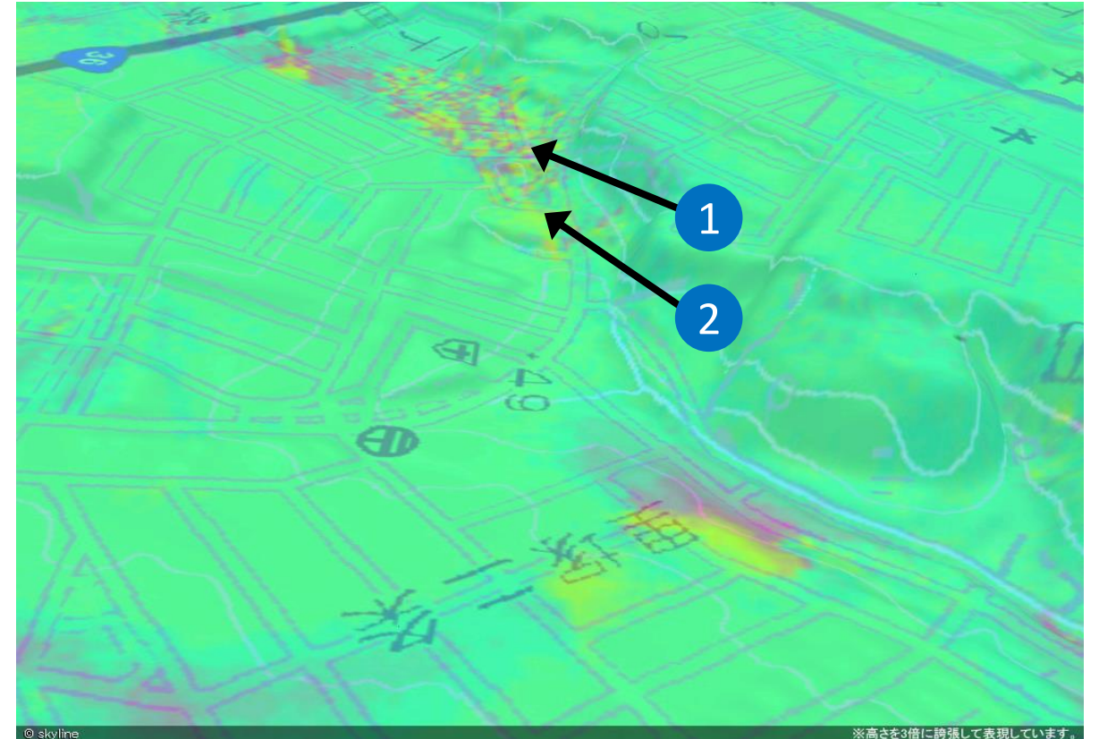
斜め写真範囲のALOS-2による地表変状抽出
